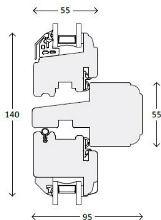
waagerechter Pfosten
