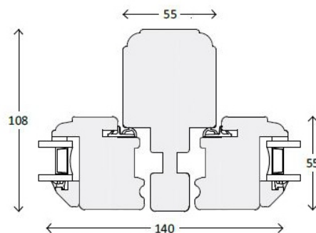
senkrechter Pfosten
